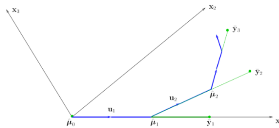
شکل شماره ۱: روال هندسی الگوریتم رگرسیون حداقل زاویه گام به گام
